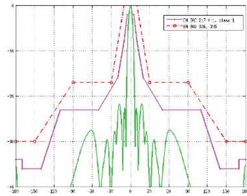
H-Plane Specs
