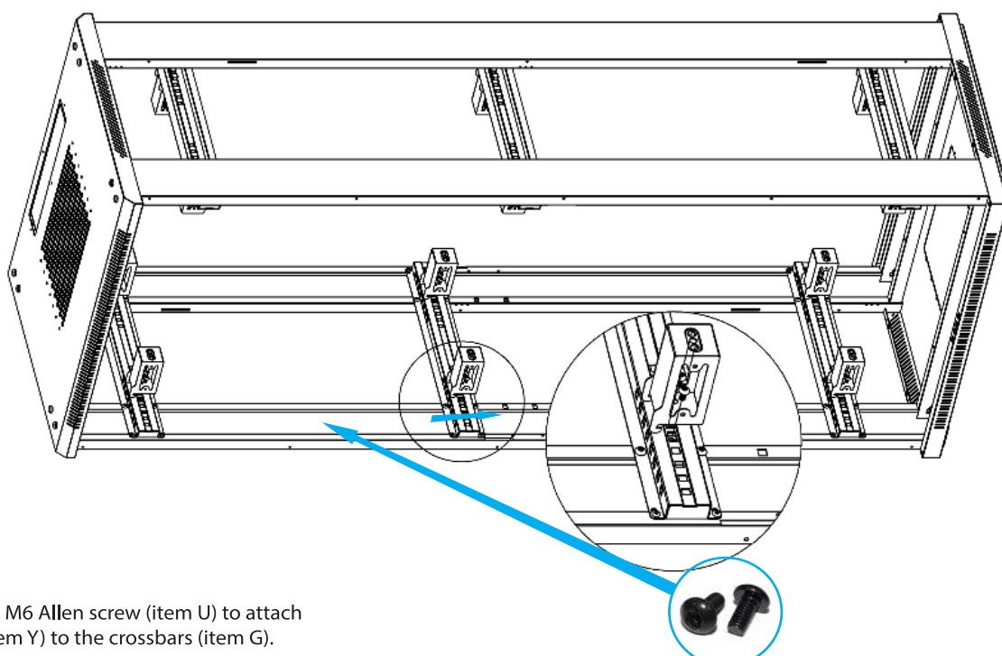
Allen head bolt M6 (part U)
