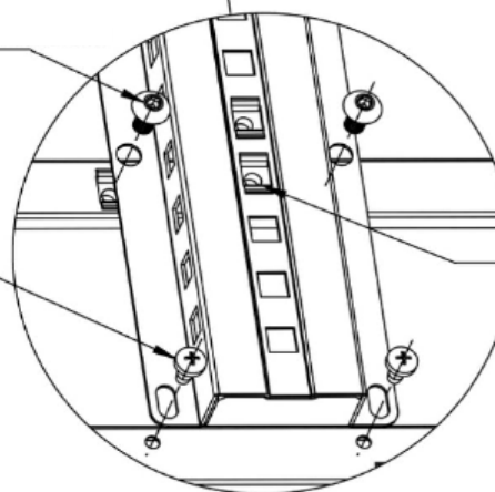
Snap nut M6 (part T)
