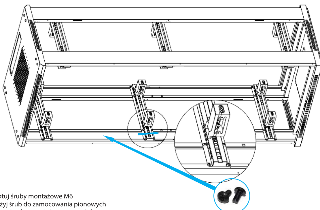
Śruba imbusowa M6 (element U)
